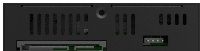
iR2771-S3 (102W × 26H × 147L mm)
